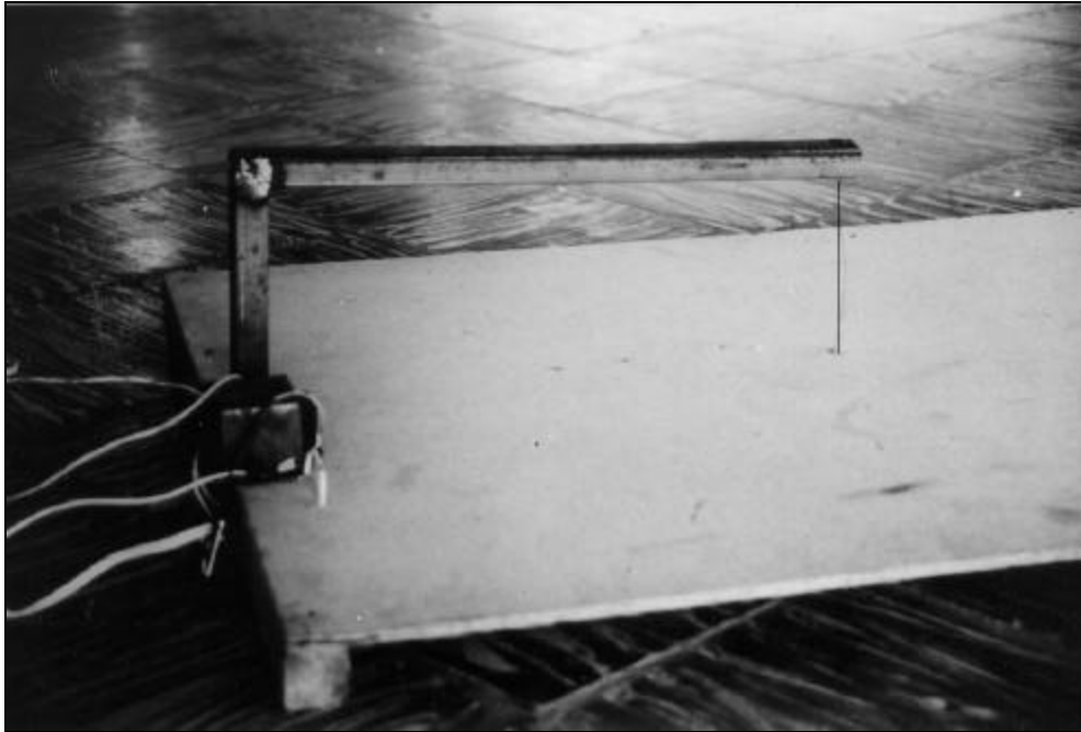
Foto 1. Cortaicopor eléctrico.
