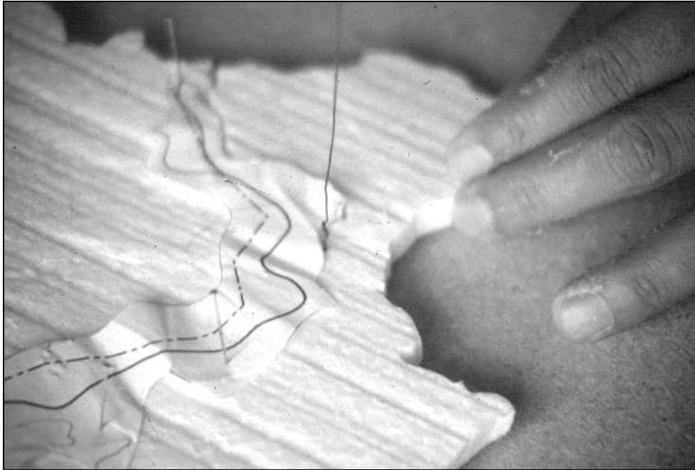
Foto 4. Corte con alambre caliente según guía de zonas de altura.
